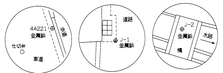
準拠点詳細図
